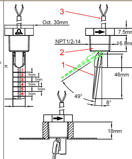
1: 柴叶 2: 主体 3: 电缆 R1F ( \frac{1}{2} " NPT)
