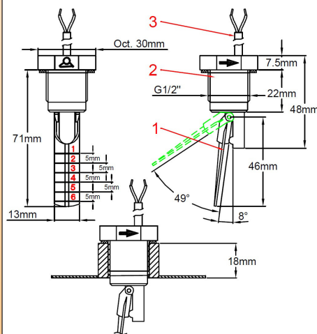
1: 柴叶 2: 主体 3: 电缆 R1S ( \frac{1}{2} " BSPP)
