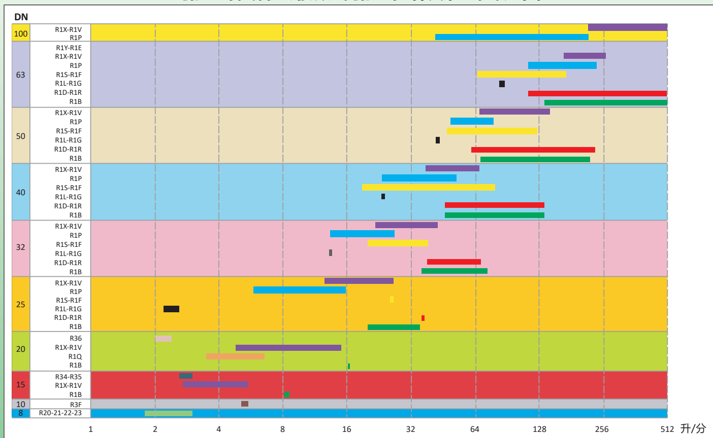
流量开关探测极限对流量和管内径的对比图
